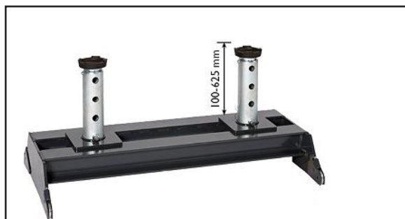
Podpora wspierająca - AB - udźwig do 20 t
